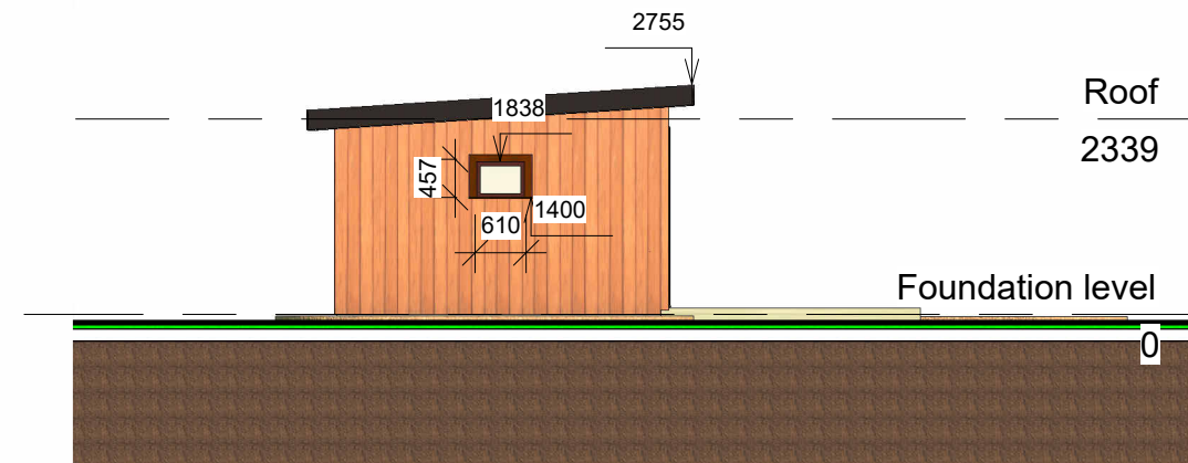
5 West 1 : 100
