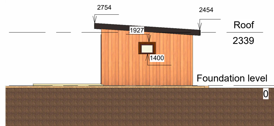
2 East 1 : 100
