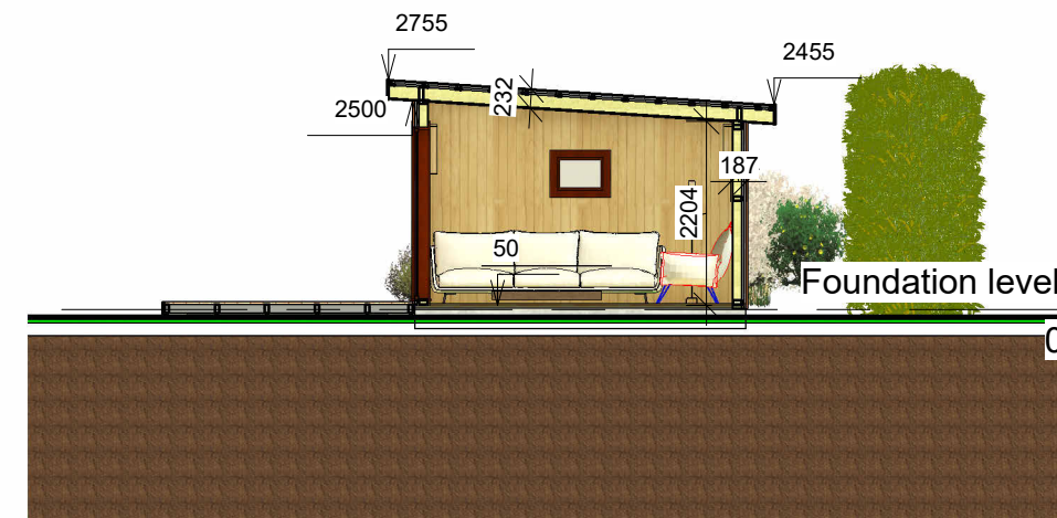
6 Section 1 1 : 100
